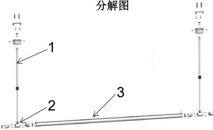
组合图
