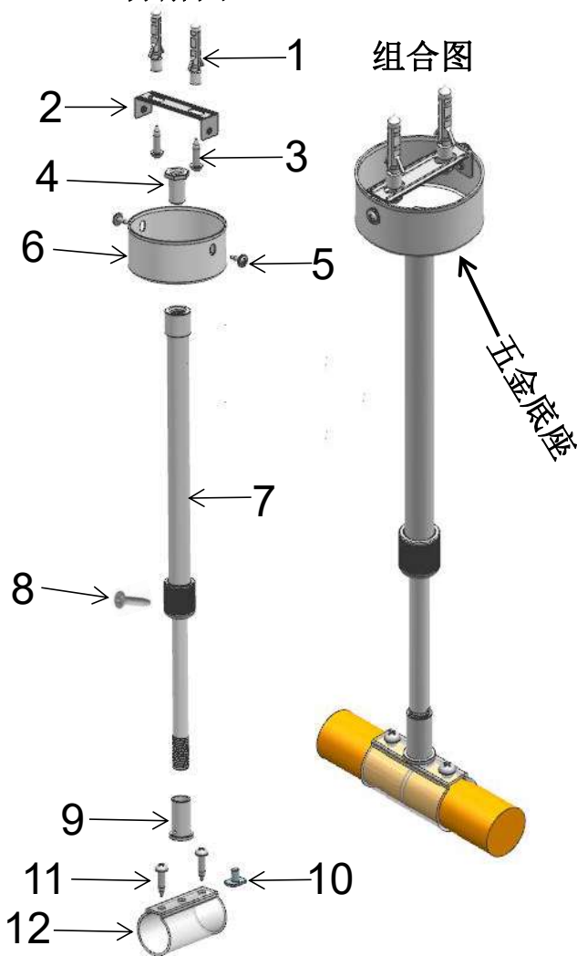
分解图
