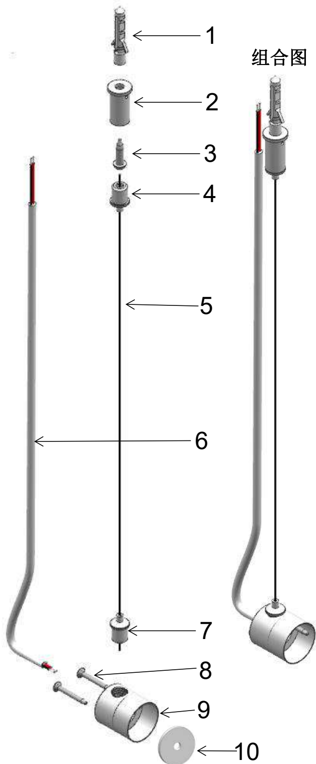
分解图
