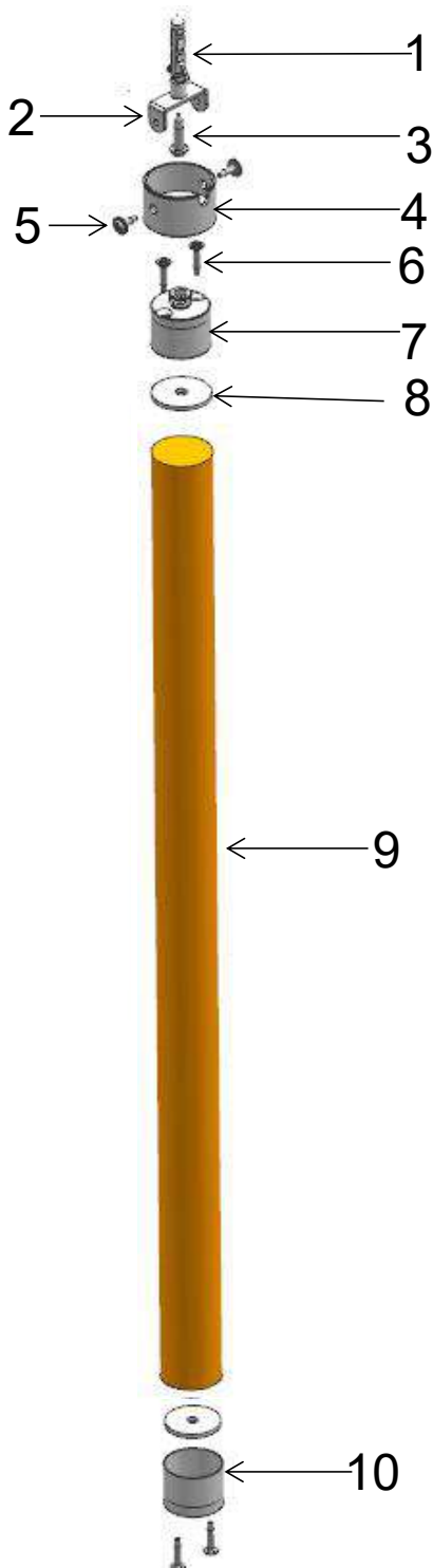
分解图
