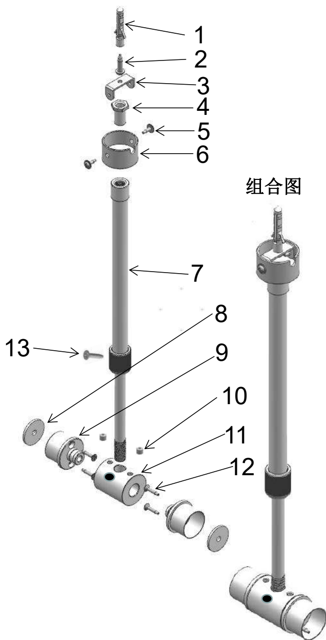
分解图
