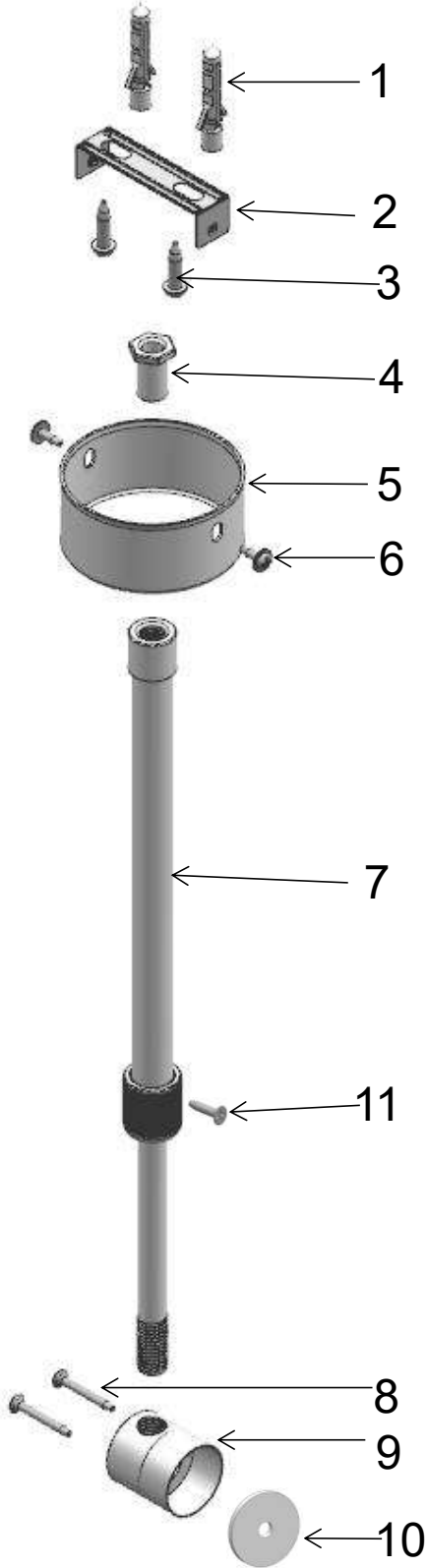
分解图
