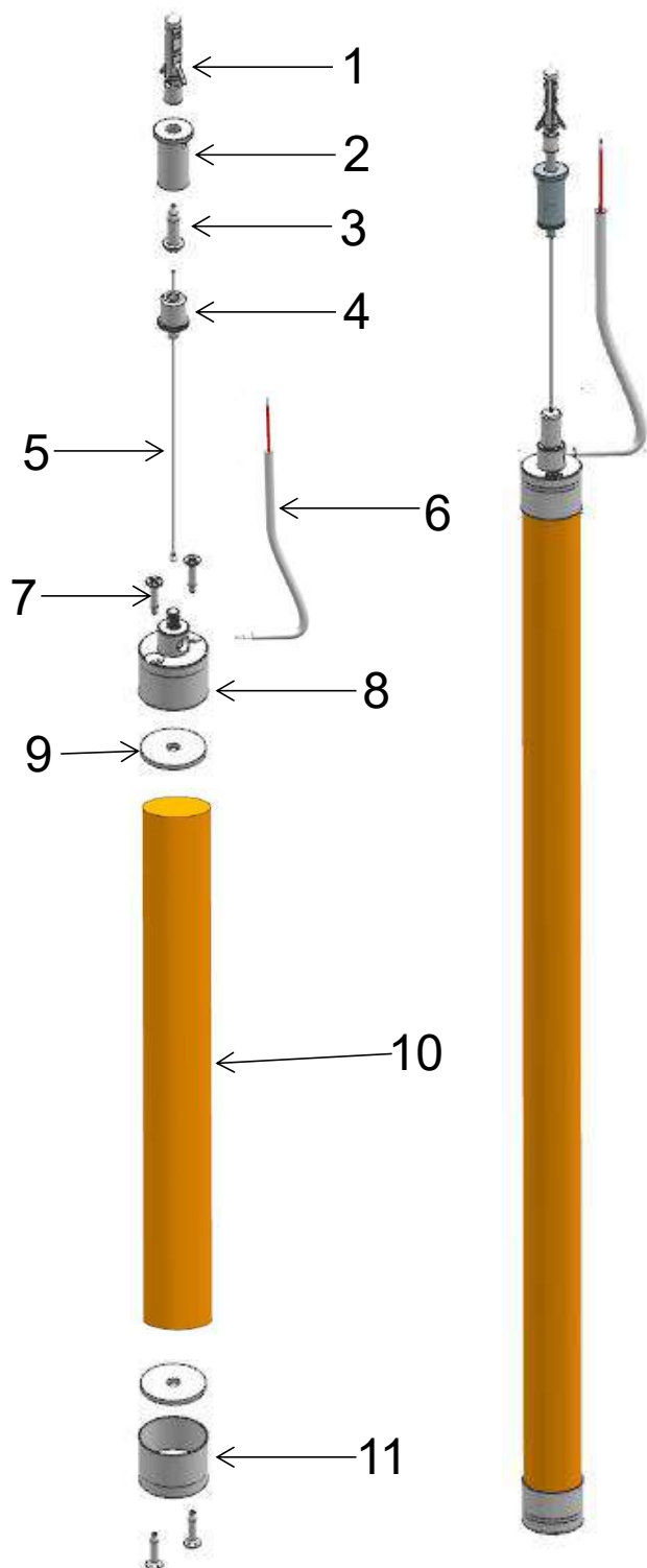
分解图
