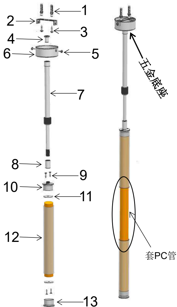
分解图
