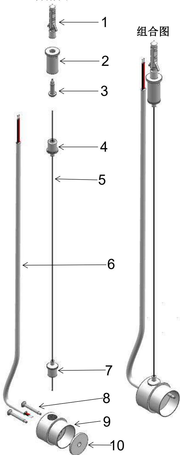
分解图
