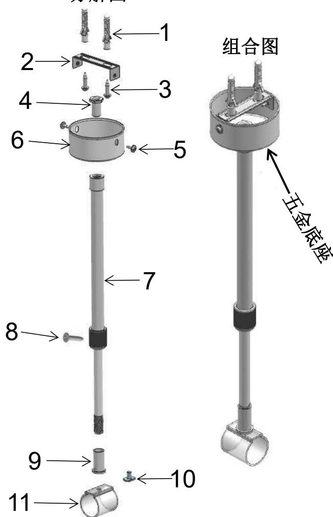
分解图
