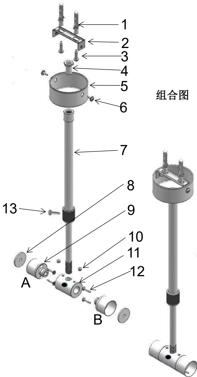
分解图
