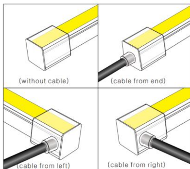
Cable outlet
